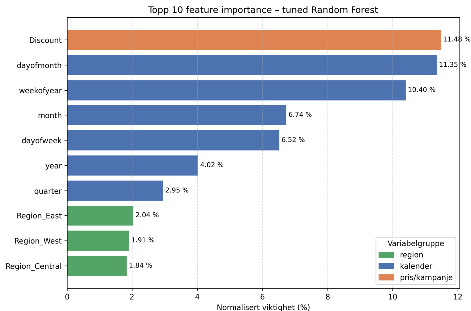
Figur 8.2 Topp 10 feature importance for tuned Random Forest. Variablene er rangert etter normalisert viktighet og viser hvilke signaler modellen faktisk vektlegger.
